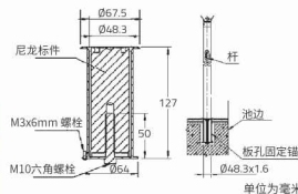
板孔固定锚 S316
