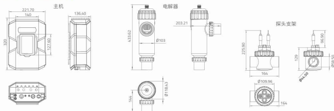
产品信息及尺寸:
