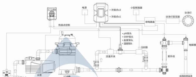
安装图
