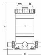
型号: CLL50 & CLL-75(硬管)
