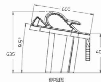
侧视图
