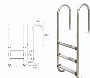
法兰不锈钢踏板
