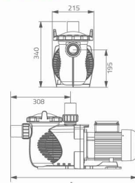
型号: SPH 水泵
