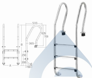
预埋件不锈钢踏板
