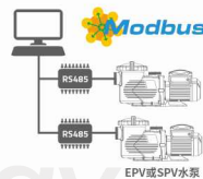
EPV或SPV水泵
