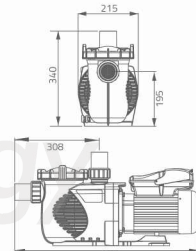
型号: SPH 2速泵
