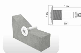
吸入管接头
