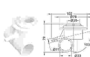
φ10&25mm水嘴身
