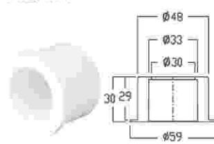
大管堵头
