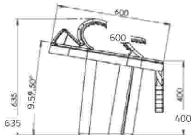
侧视图
