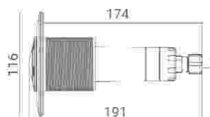
吸入管接头
