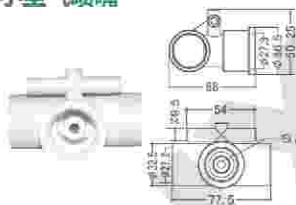
小型气喷嘴
