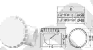
φ2寸L型截面排水口 (滑入型)
