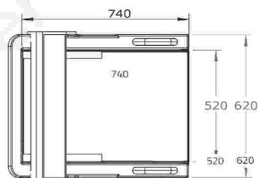
俯视图
