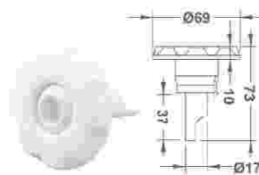
φ2-3/4寸球型水疗喷嘴
