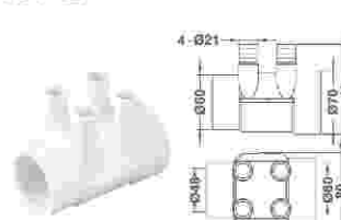
分水管
