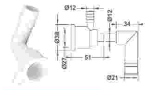
L型暗嘴身
