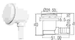
单孔气嘴
