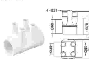
分水管
