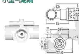
小型气喷嘴
