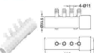
分气管
