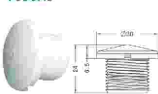
单孔喷嘴
