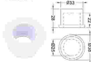
小管堵头
