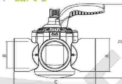
FLEX 3通阀
