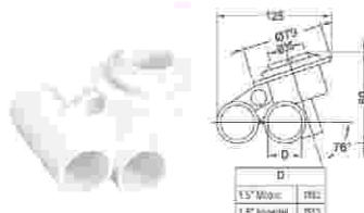
φ25mm T型喷嘴身
