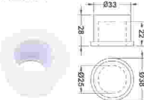
小管堵头
