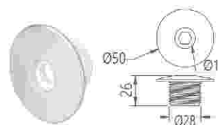
光面喷嘴
