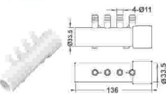
分气管
