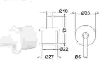
小管堵头
