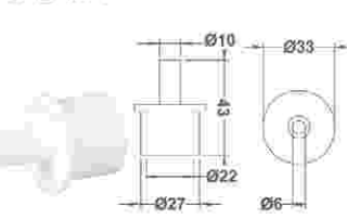
小管堵头
