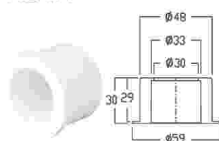
大管堵头
