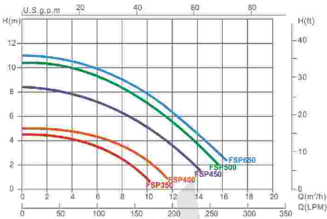
注：以上性能曲线为50Hz型号
