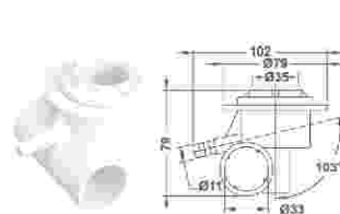
φ10&25mm水嘴身
