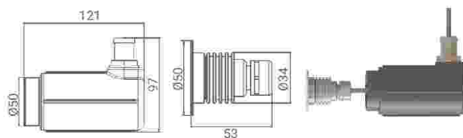
TL-1C
